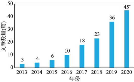
图2 使用远程耦合框架的文章数量 Fig. 2 Number of papers that used the telecoupling framework
