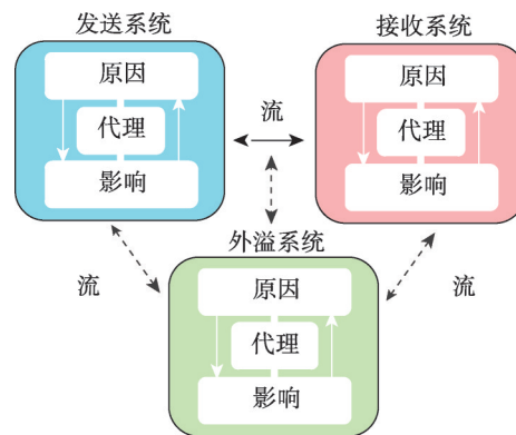
图1 远程耦合框架示意图(参考文献[14]修改)
